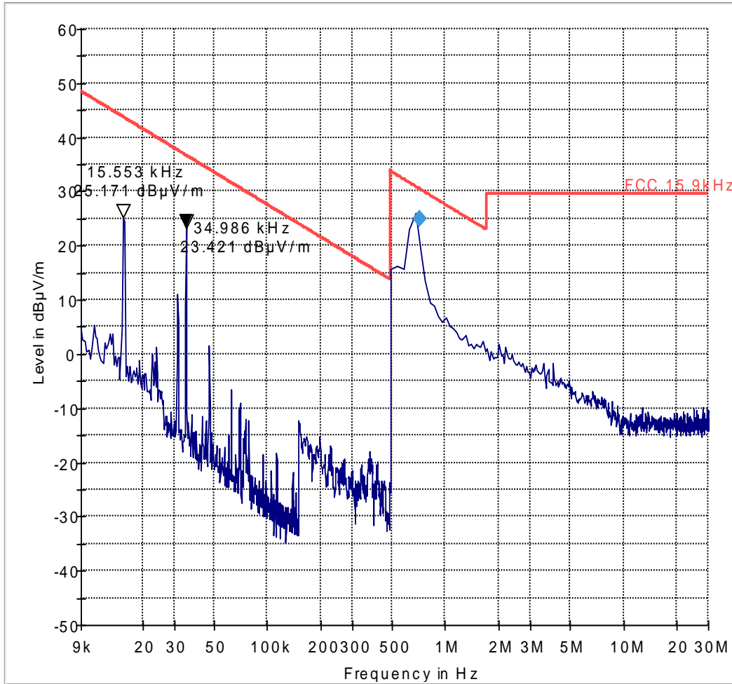
FCC 15 9kHz - 30 MHz
