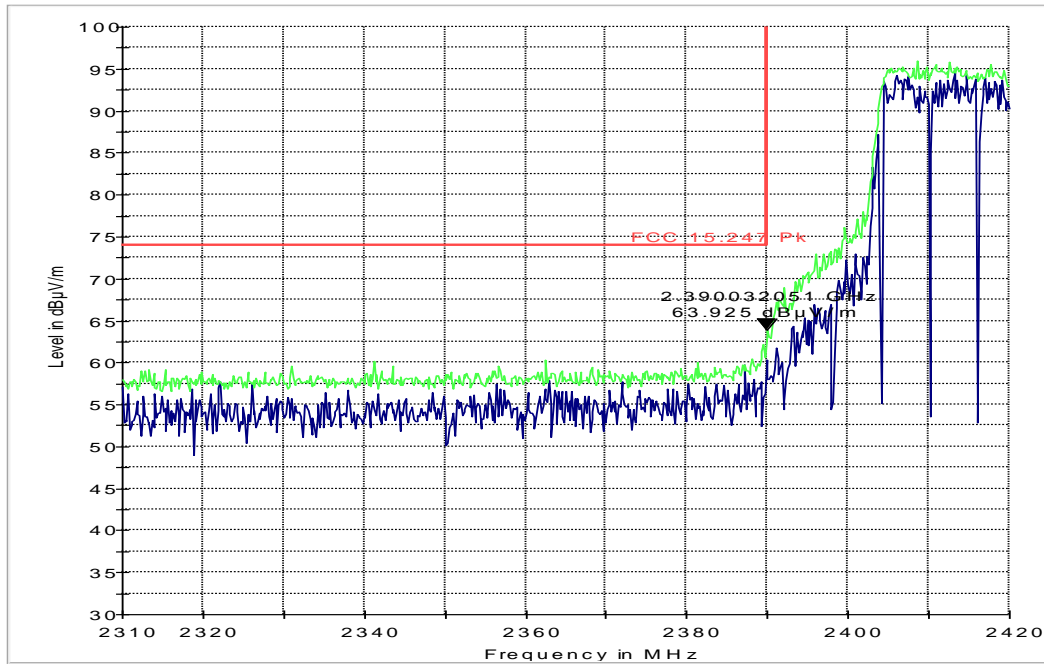
FCC 15.247 LBE Pk 3m
