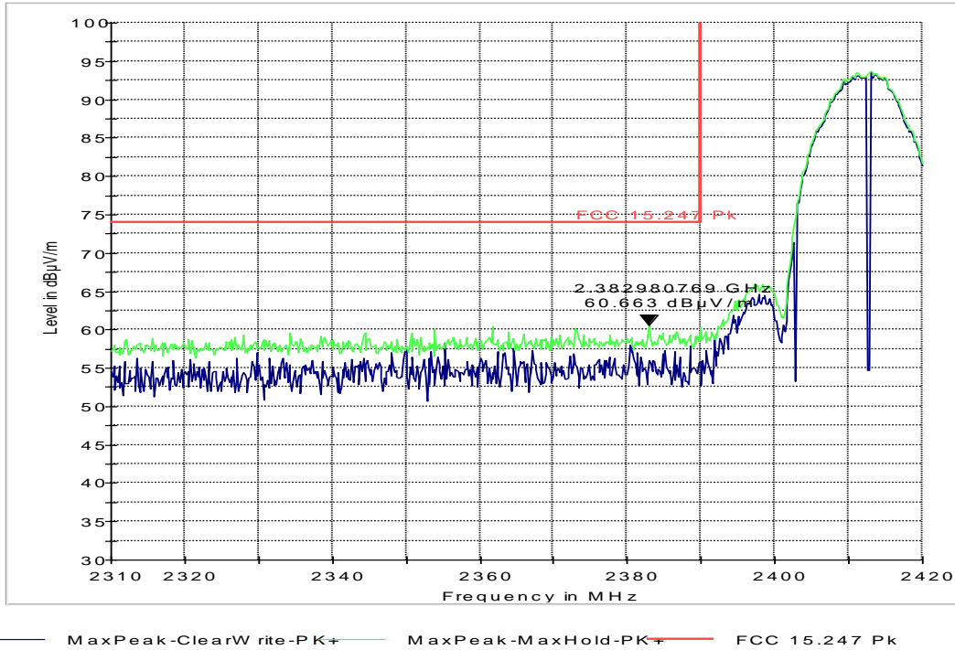
FCC 15.247 LBE Pk 3m
