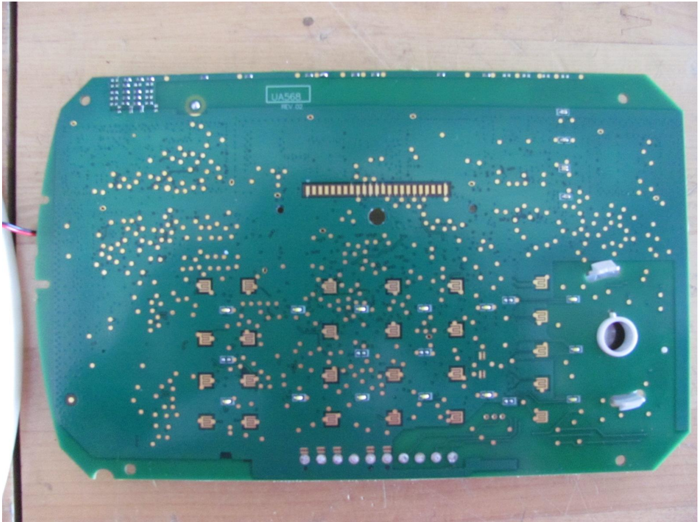
SCW9057-433 UA558 Rev 03 PCB bottom view
