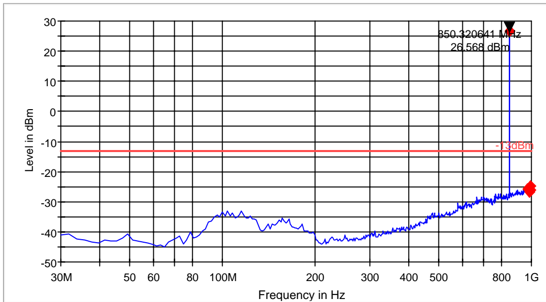
FCC 22 30-1000MHz
