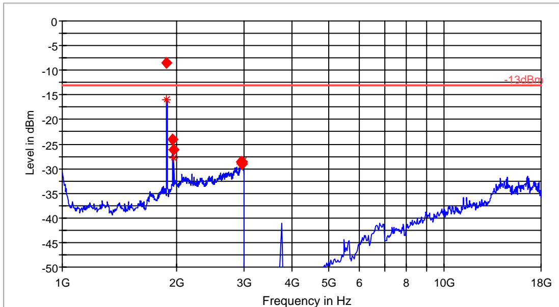
FCC 24 1-18GHz
