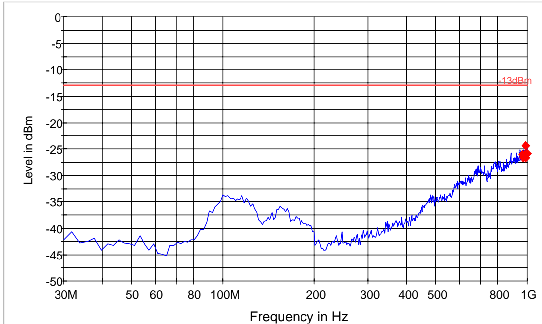
FCC 22 30-1000MHz
