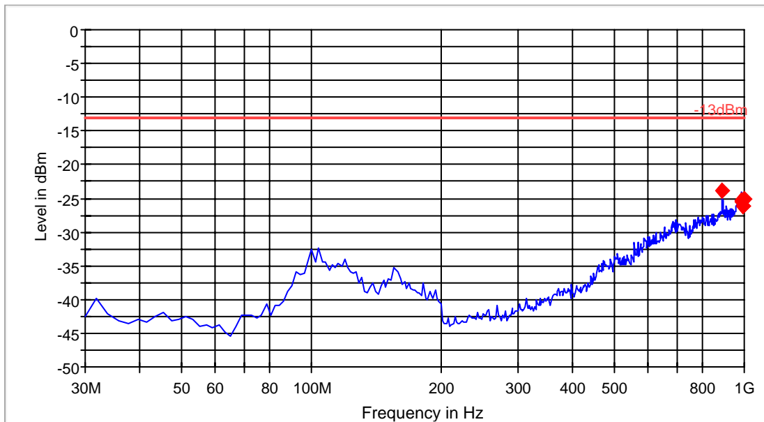
FCC 22 30-1000MHz
