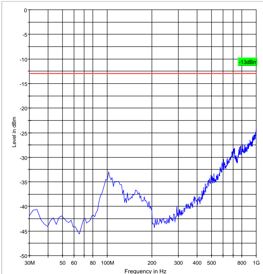
FCC 22 30-1000MHz
