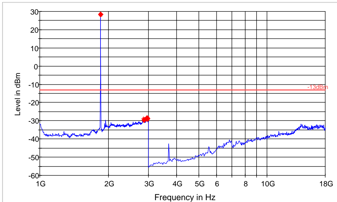
FCC 24 1-18GHz
