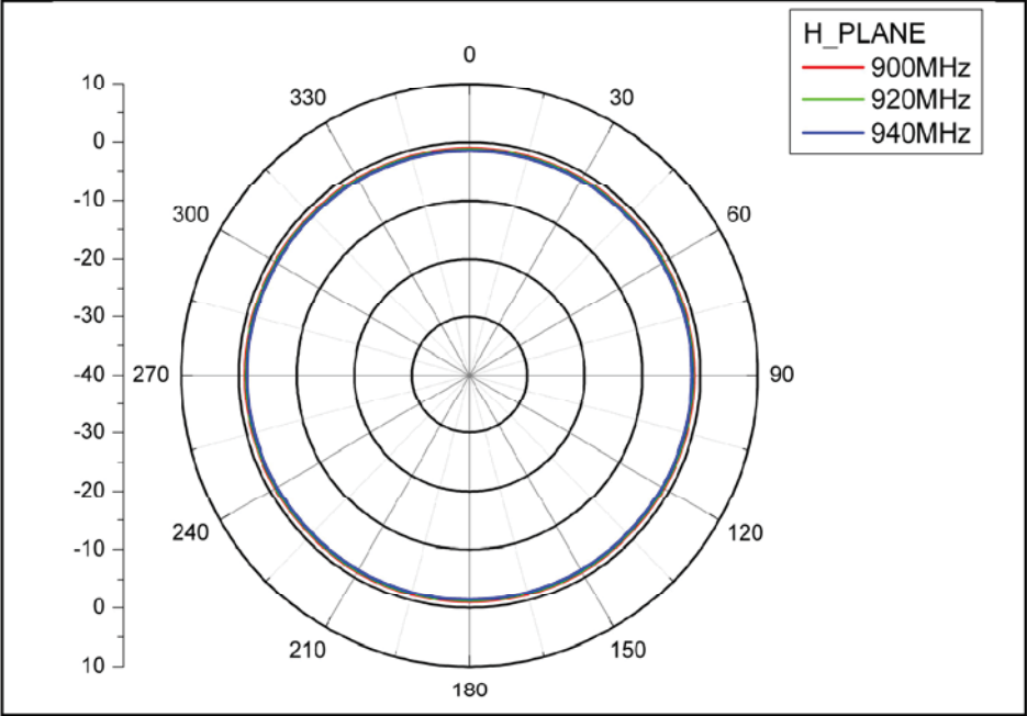
H-plane
