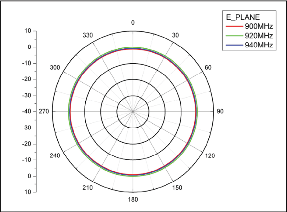
E-plane
