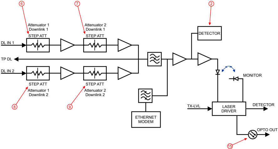
Figure 82 FOI Downlink Measurement Locations
