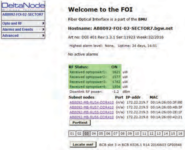
Figure 79 FOI Welcome Screen SW Version 3.9, DOI401
