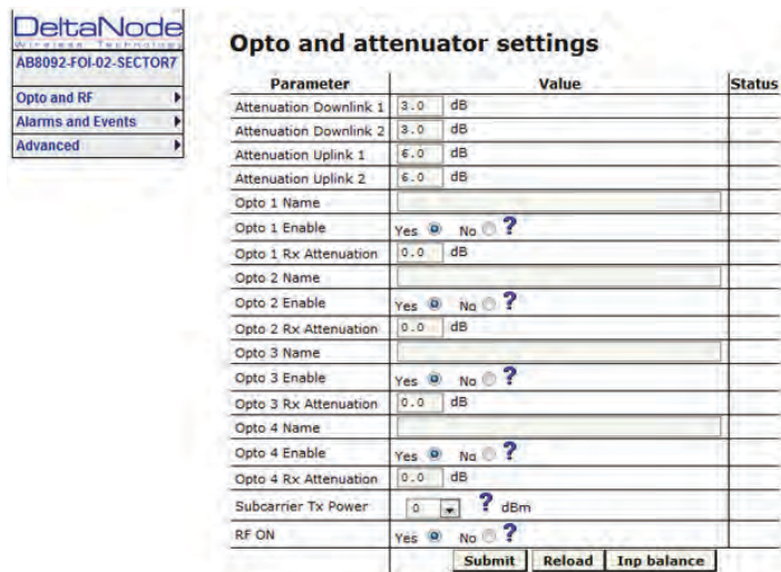
Figure 87 DOI401 FOI Opto and Attenuator Settings
