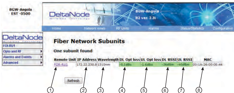
Figure 88 FOI Fiber Network Subunits
