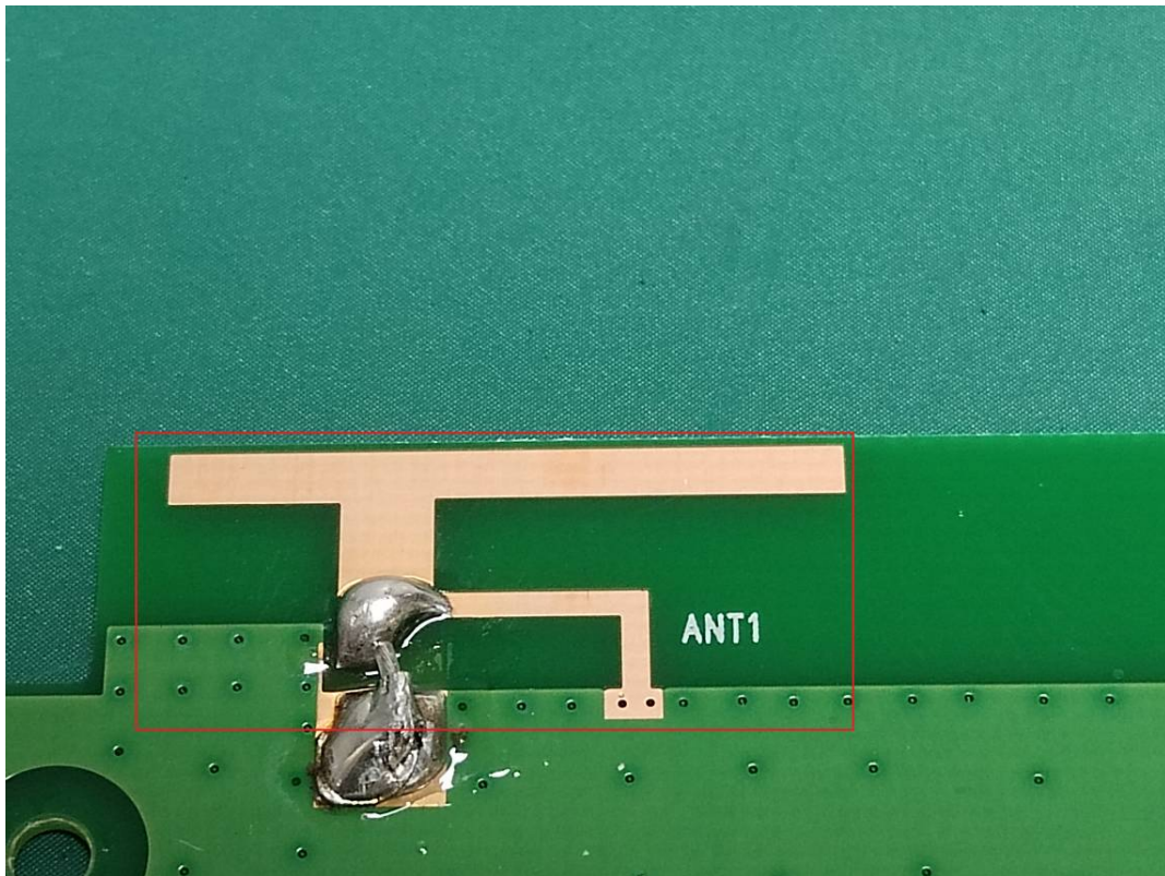
Wi-Fi ANT1
