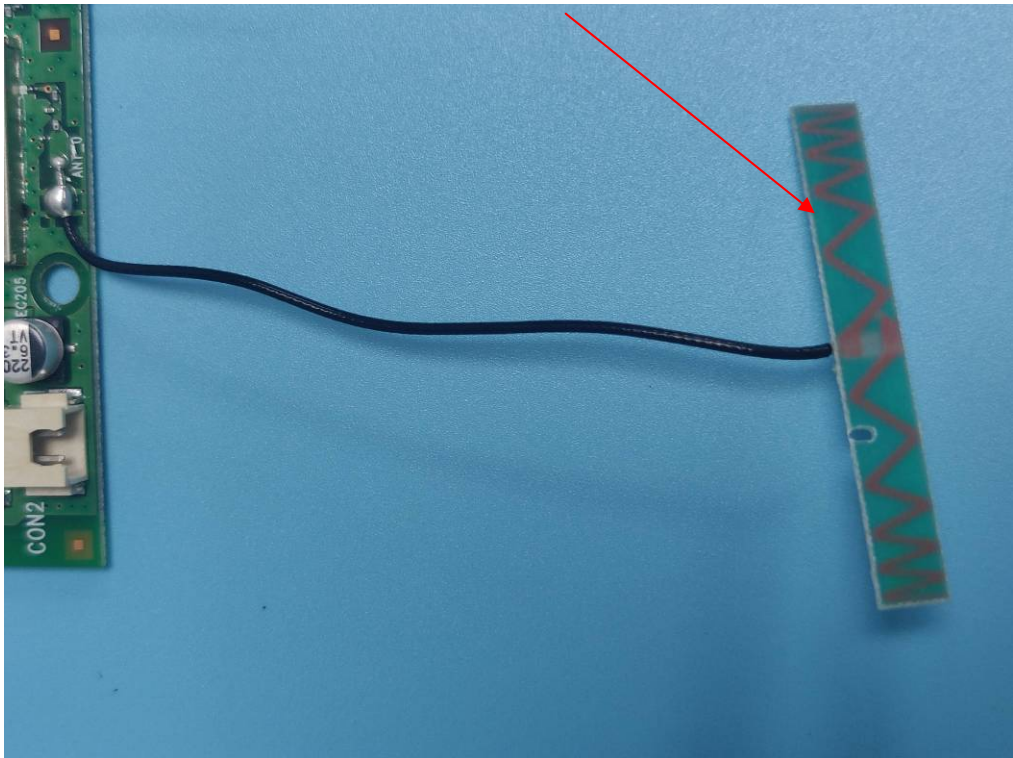
DECT ANT0
