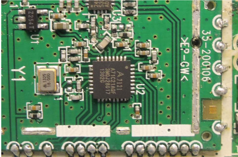
RFIC
