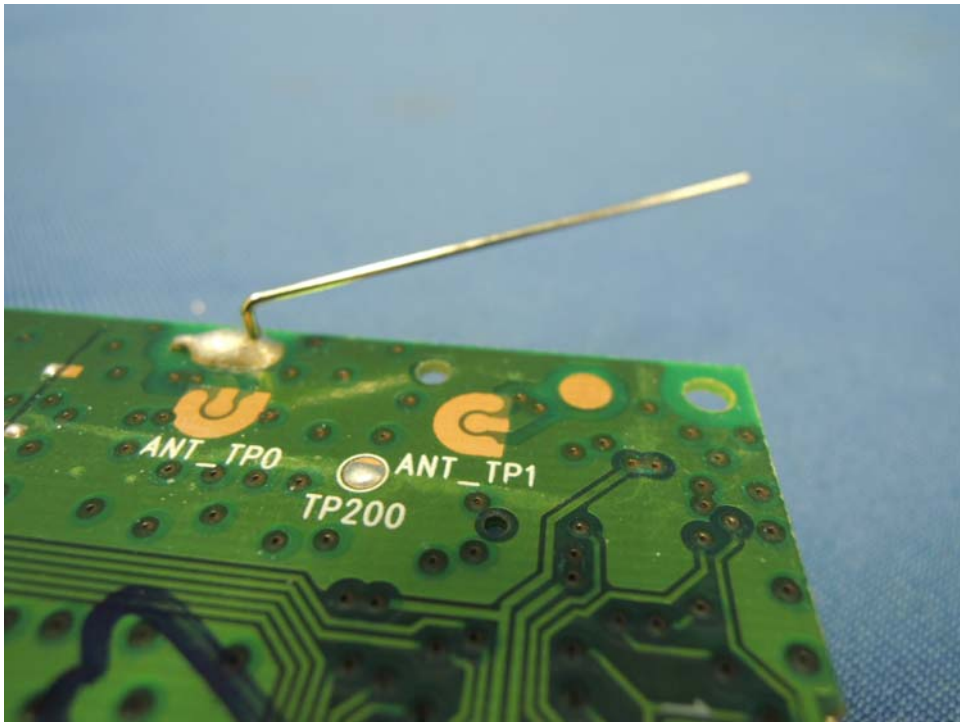
Base Unit DECT Antenna (ANT0)
