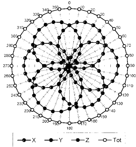
f = 600 MHz, TEM ifi110EXX
