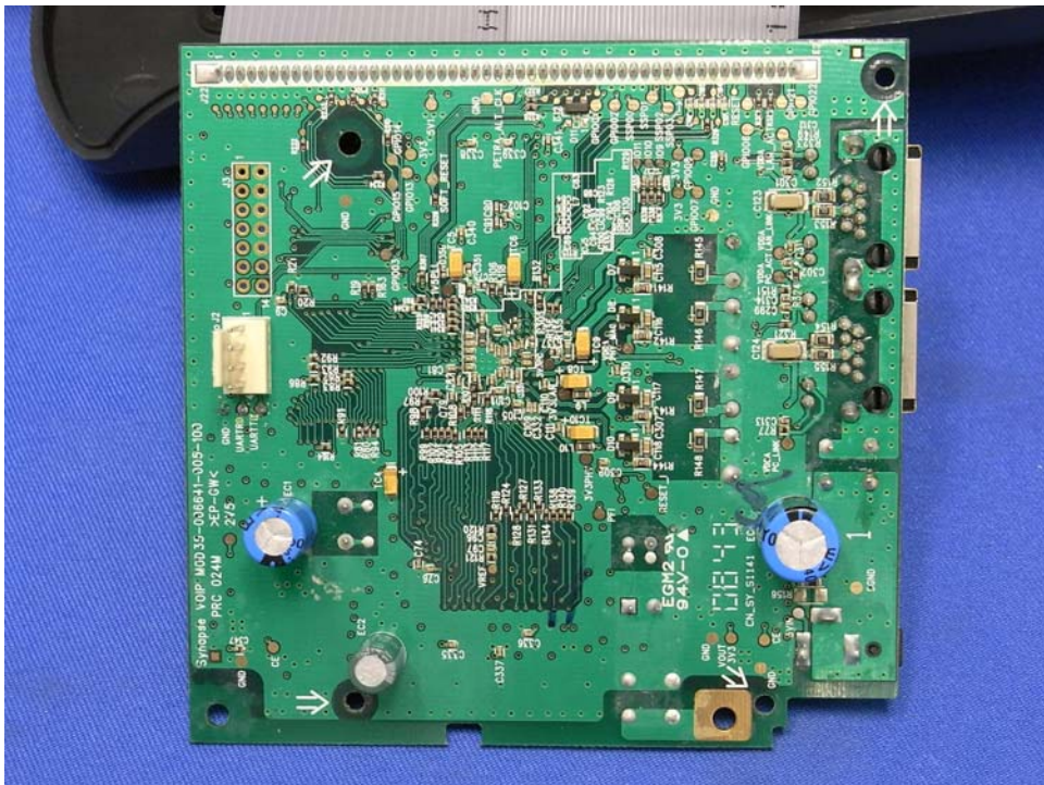
Deskset VoIP PCB rear side
