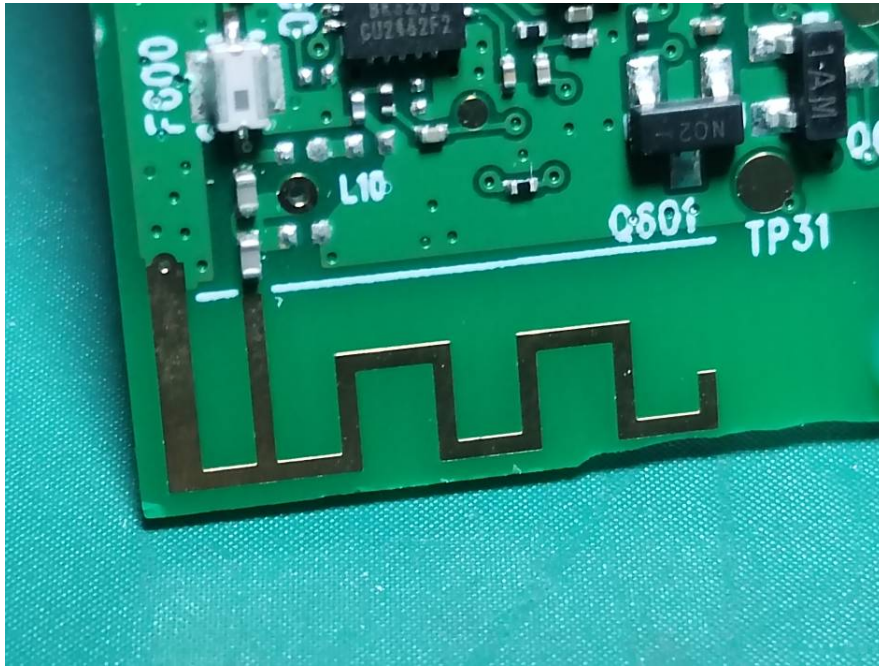
BT ANT
