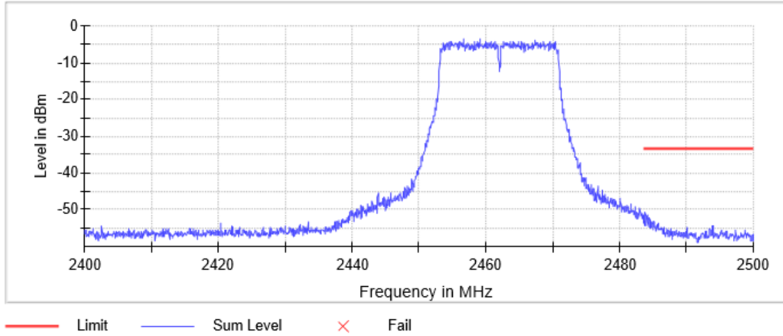
Band Edge
