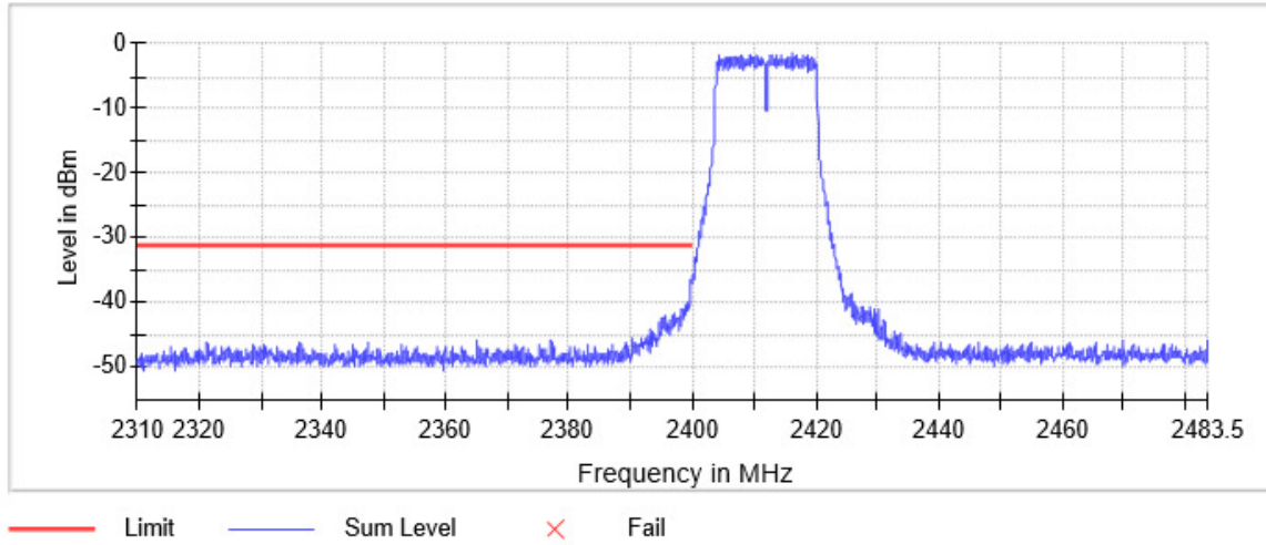
Band Edge
