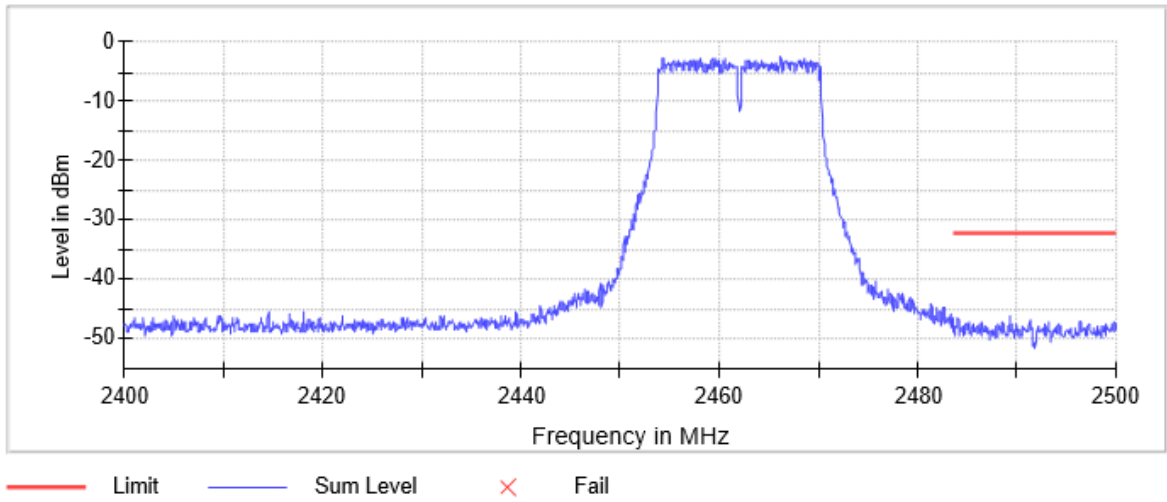
Band Edge
