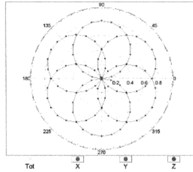
f=1800 MHz,R22
