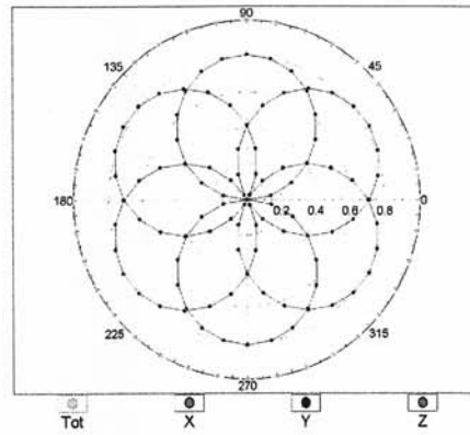
f=1800 MHz,R22
