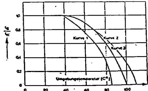
Kurve 1: max. Betriebstemperatur 85° I 0 : max. Betriebsstrom Kurve 2: max. Betriebstemperatur 100°C I 0 : Nennstrom bei Umgebungstemperatur +40°C Kurve 3: max. Betriebstemperatur 110°C
