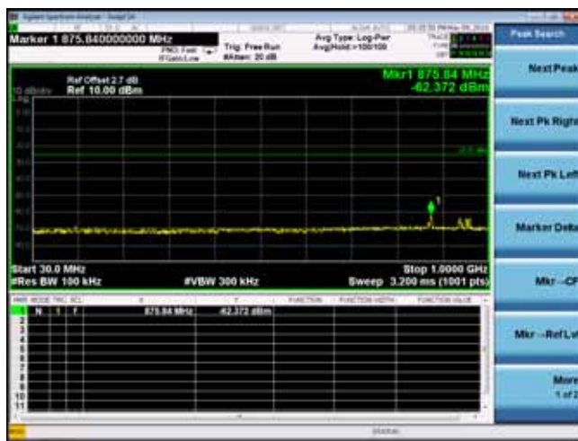
2480MHz(30MHz – 1GHz)
