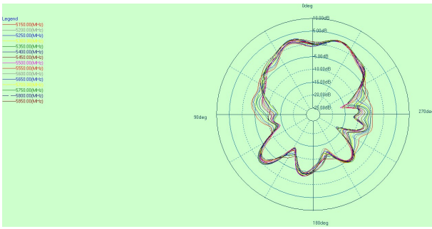
5G phi=0deg
