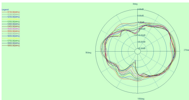
5G theta=90deg
