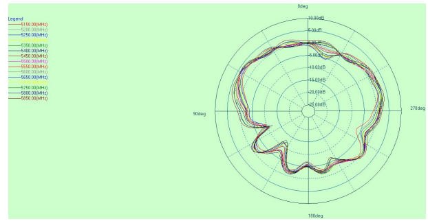
5G phi=90deg
