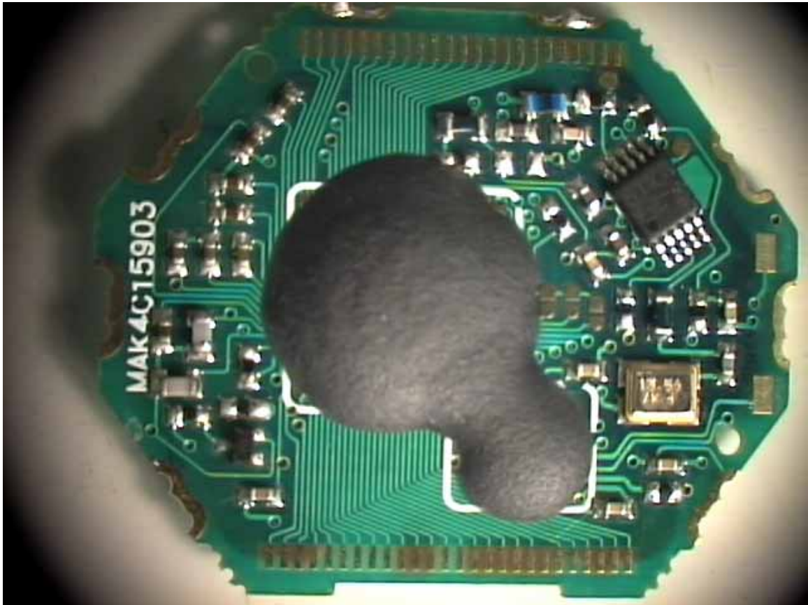
PCB (display side)
