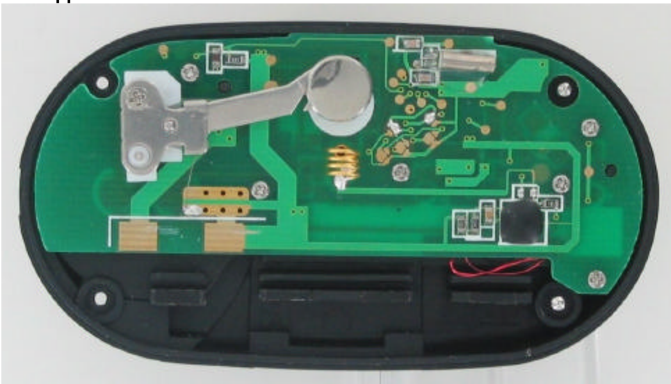
Antenna
