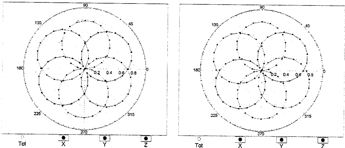
f=1800 MHz,R22
