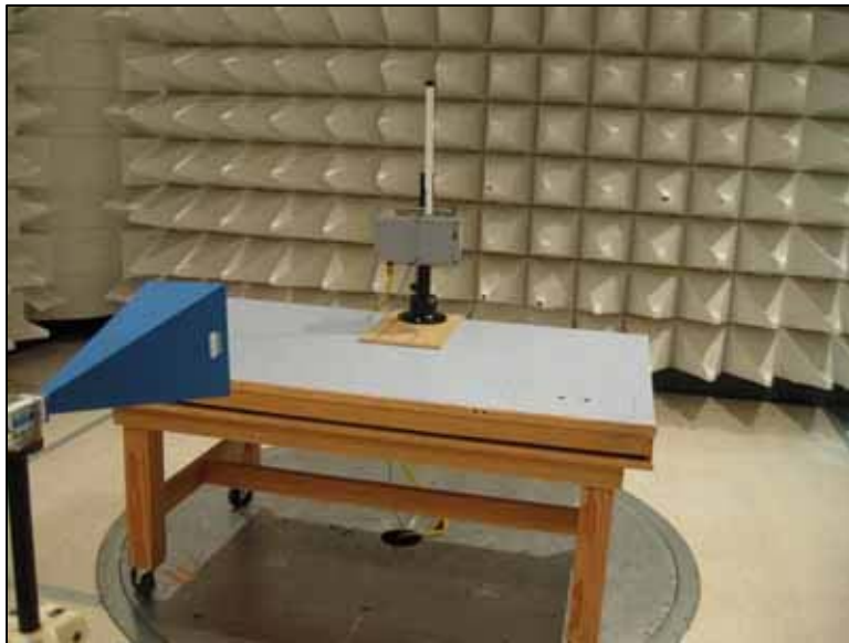
10-18GHz CCU100B
