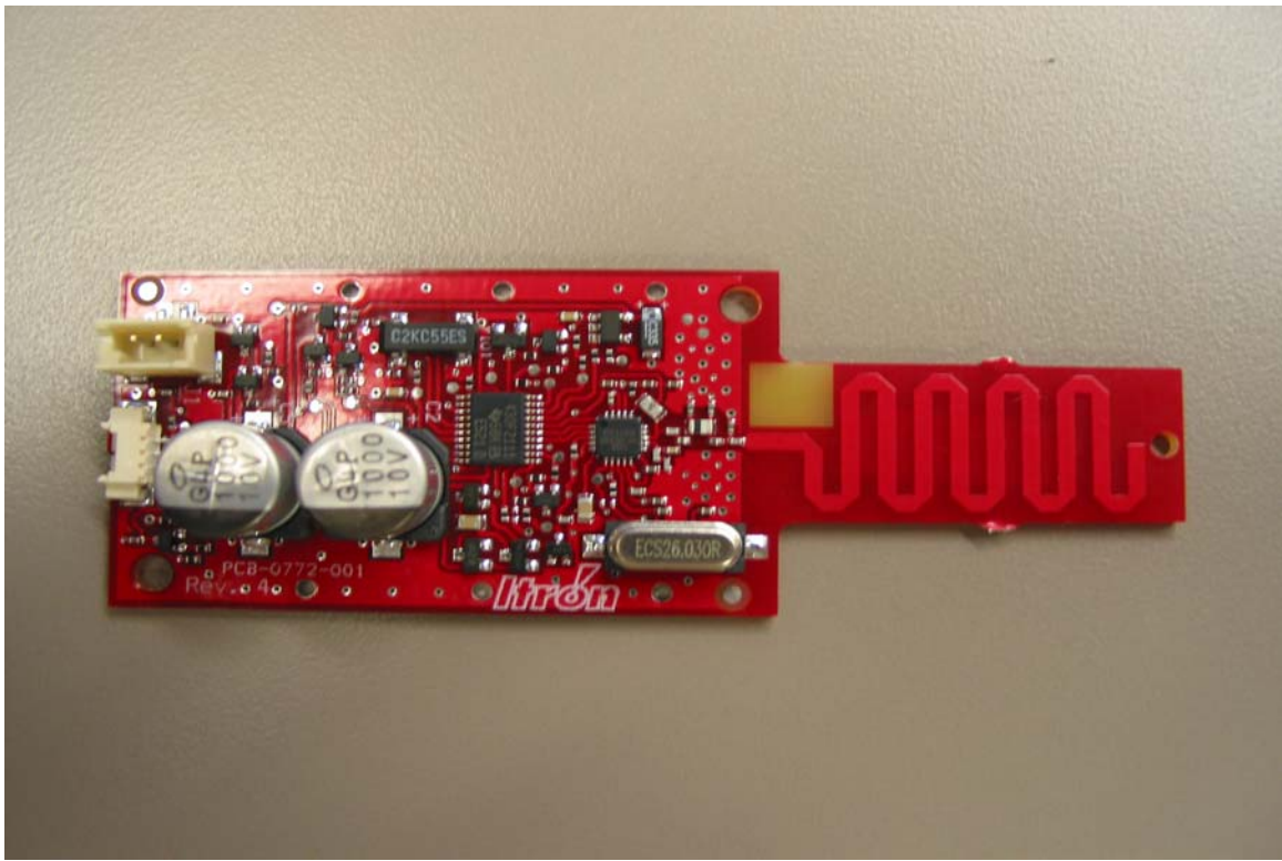
Figure 1 PCA Top
