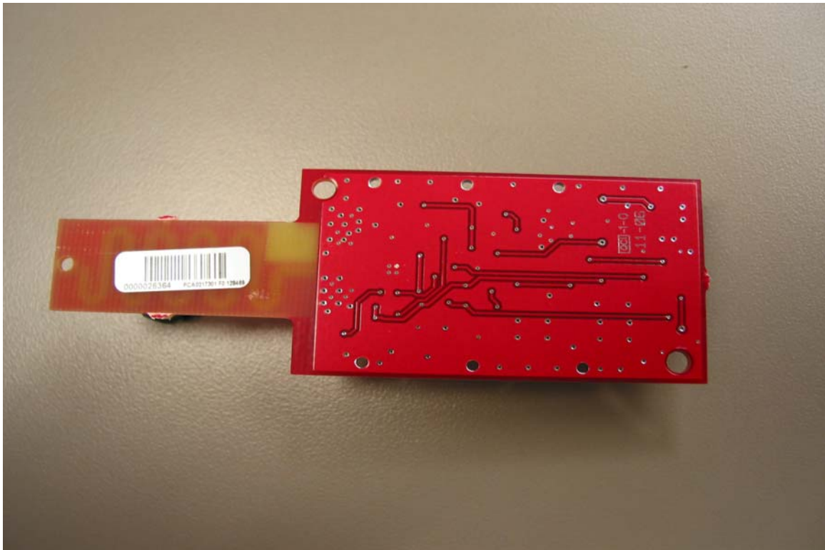
Figure 2 PCA Bottom
