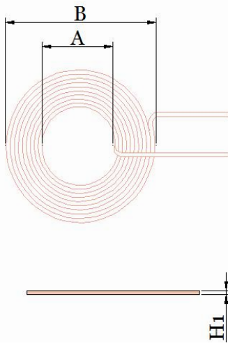
图一、线圈
