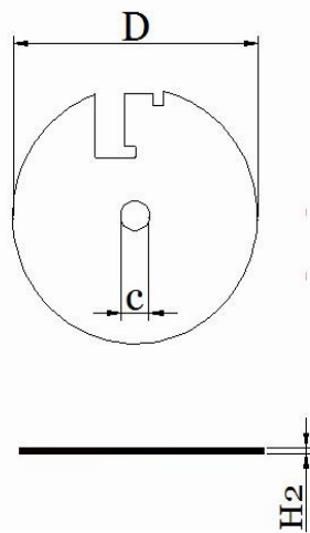
图二、硬磁片
