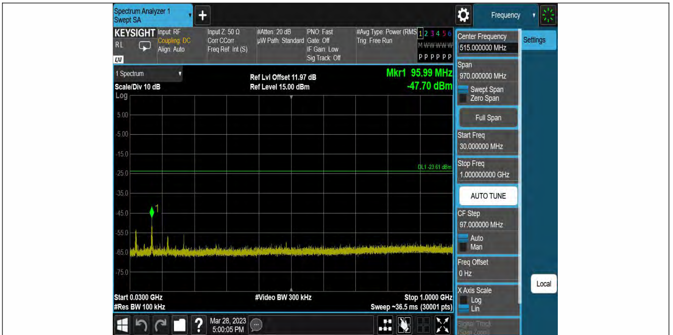
DH5-Ant1-2441-30~1000--3.61
