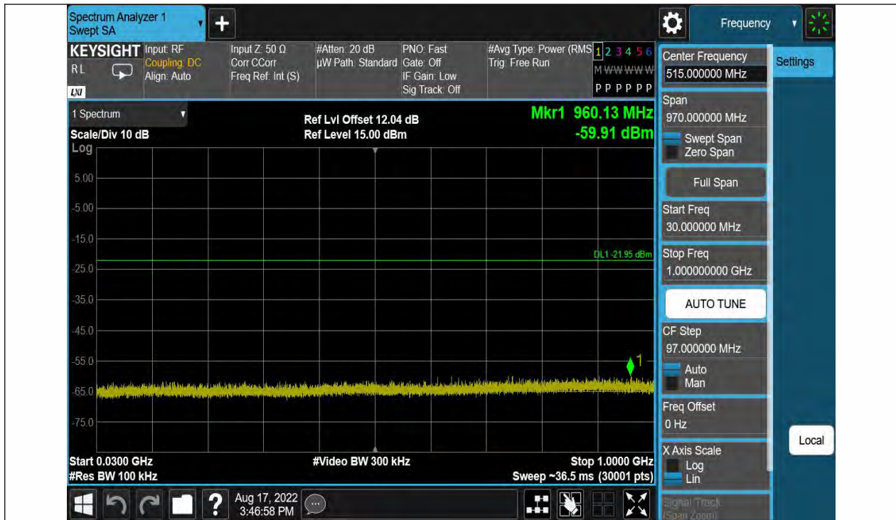
BLE 1M Ant1 2440 30~1000
