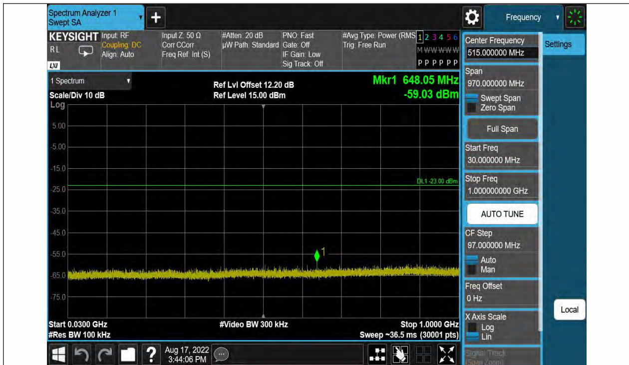
BLE 1M Ant1 2402 30~1000
