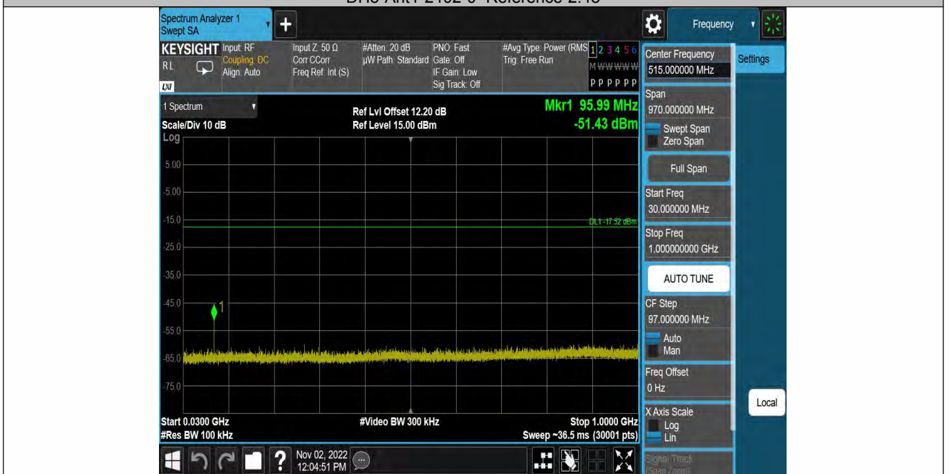
DH5-Ant1-2402-30~1000-2.48
