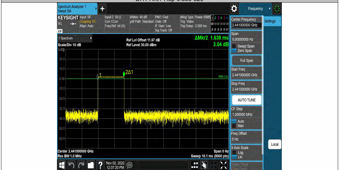
DH3-Ant1-Hop-1.638-160
