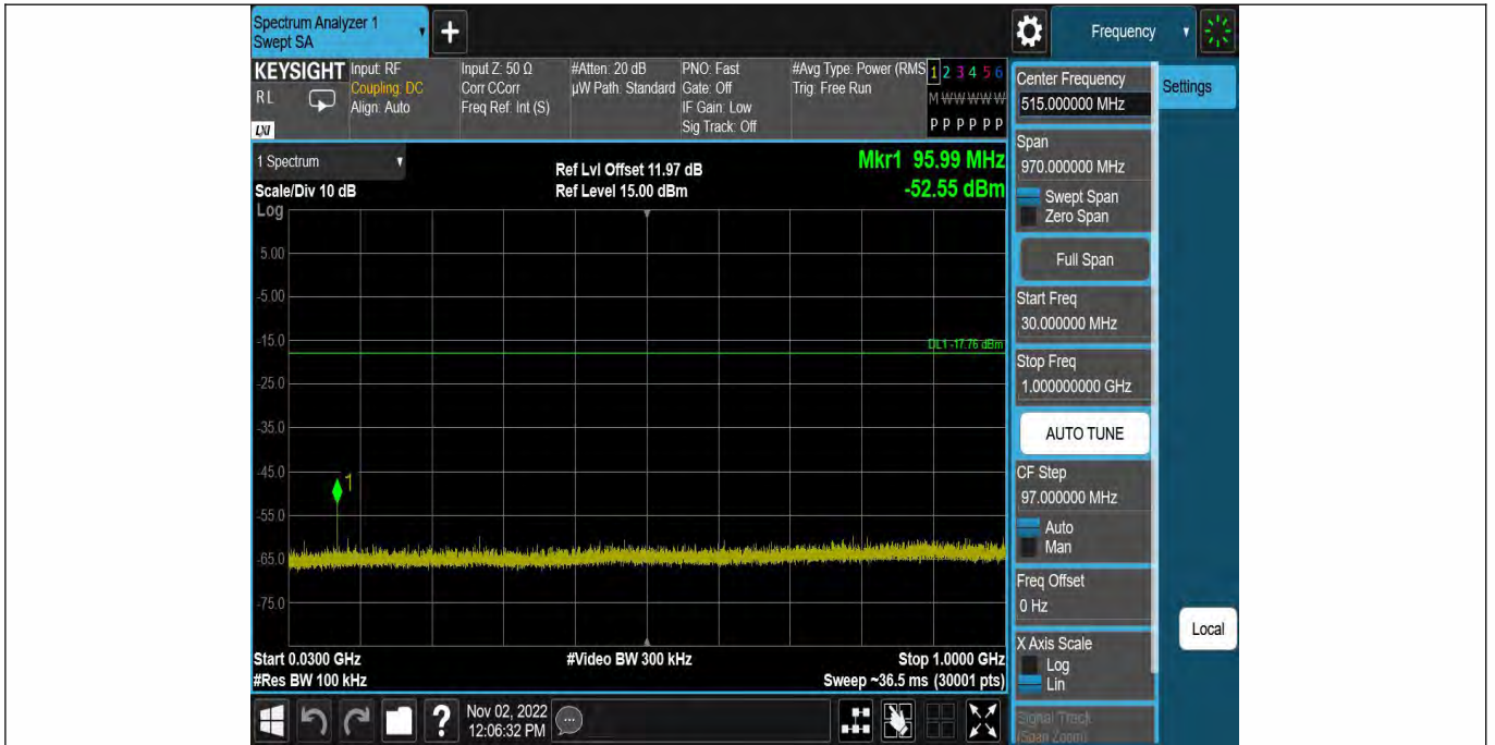
DH5-Ant1-2441-30~1000-2.24
