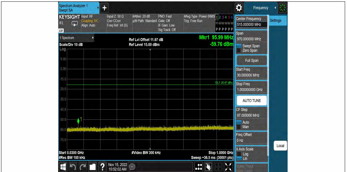
DH5-Ant1-2441-30~1000--0.47
