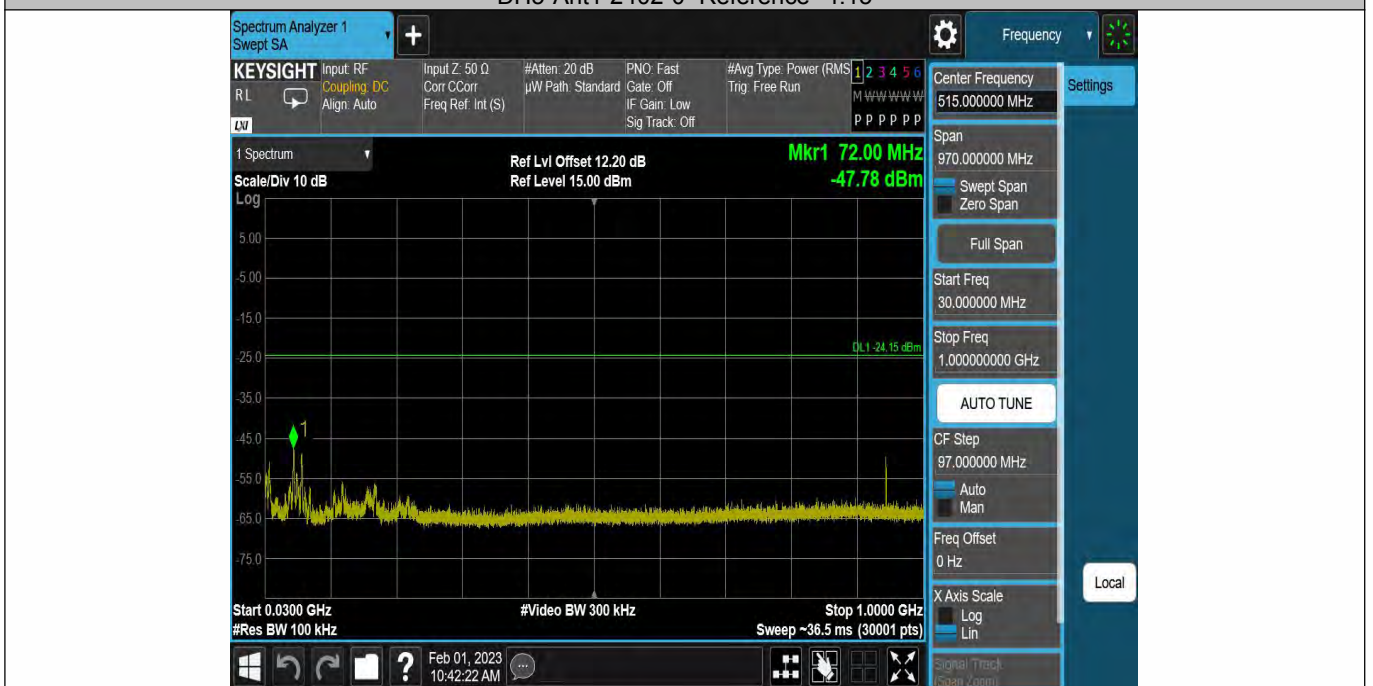
DH5-Ant1-2402-30~1000--4.15
