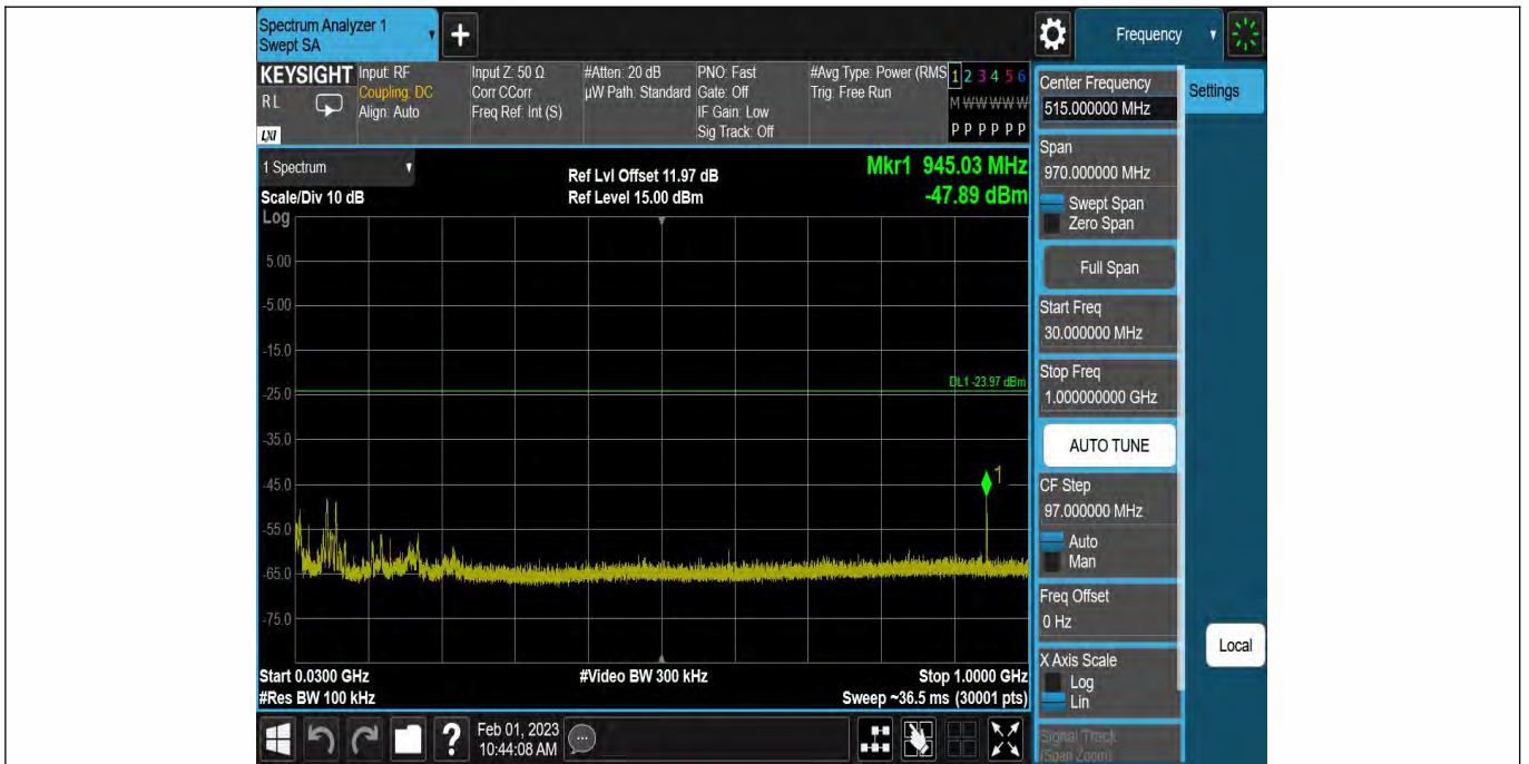
DH5-Ant1-2441-30~1000--3.97
