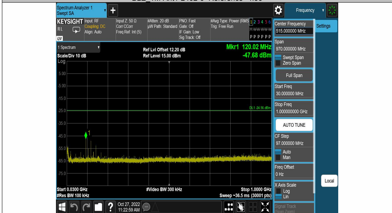
BLE 1M-Ant1-2402-30~1000--4.56
