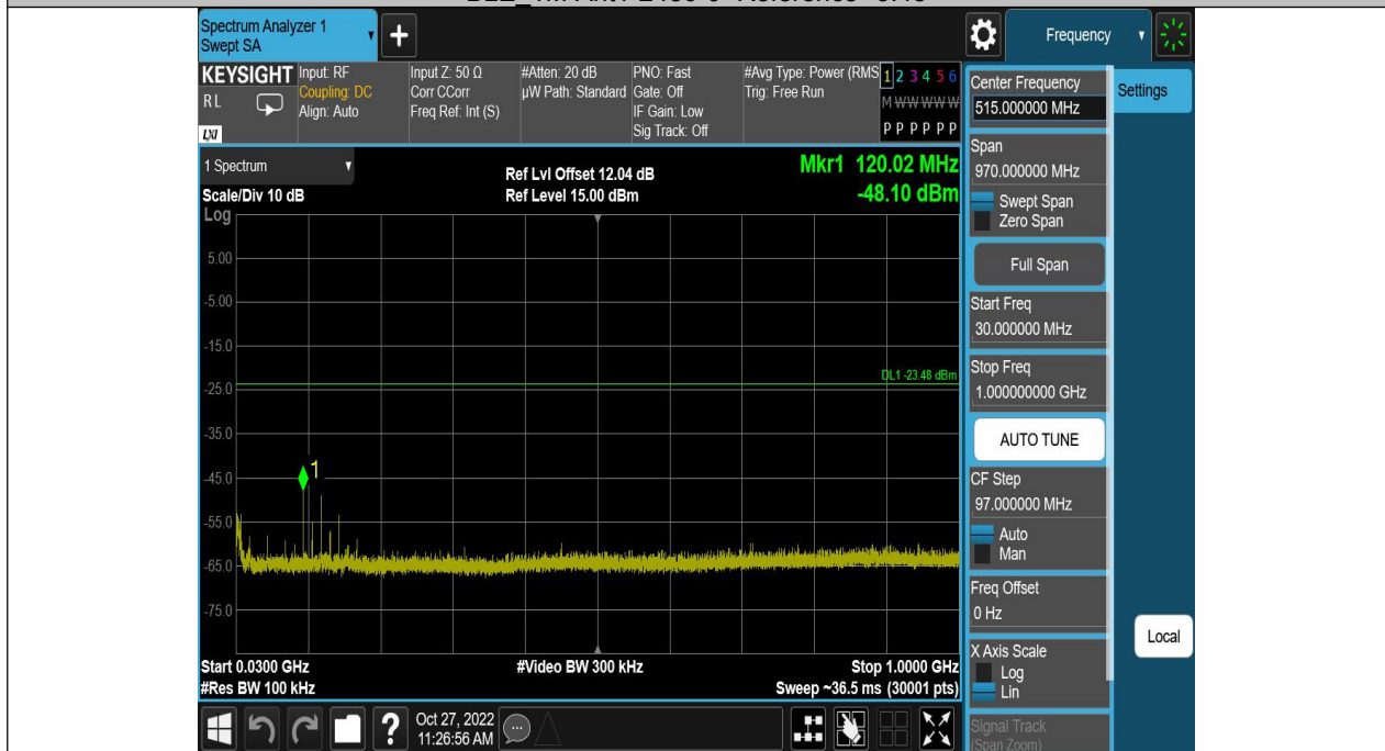
BLE 1M-Ant1-2480-30~1000--3.48
