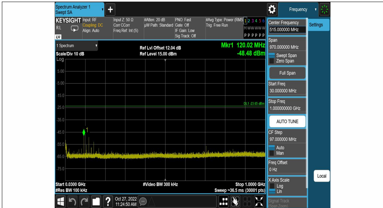
BLE_1M-Ant1-2440-30~1000--3.65
