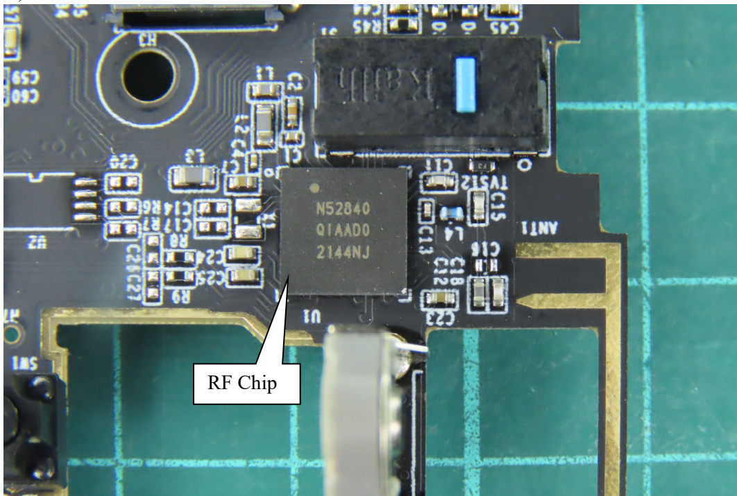
(12) EUT Photo
