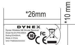
DX-PWLMSEA Dongle label SCALE: 1:1
