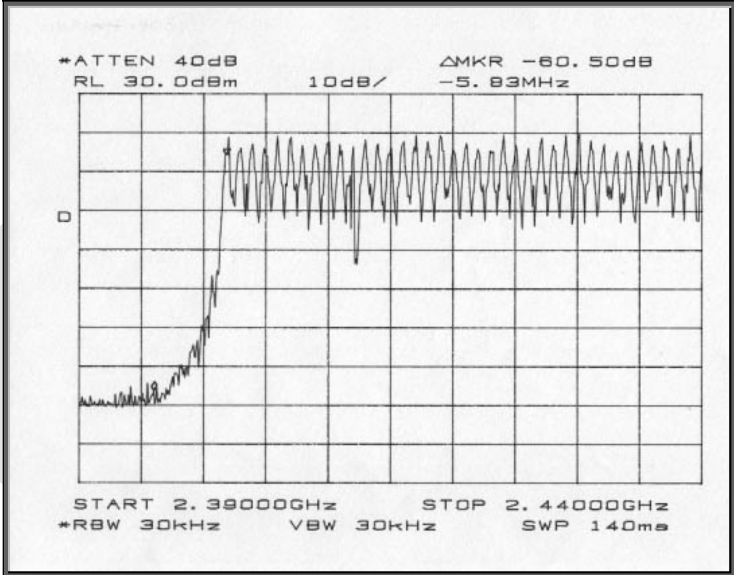
Lower Band Edge
