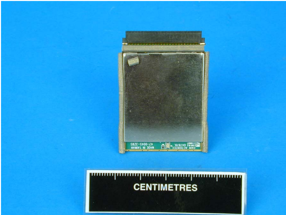
Top view, 802.11b radio module
