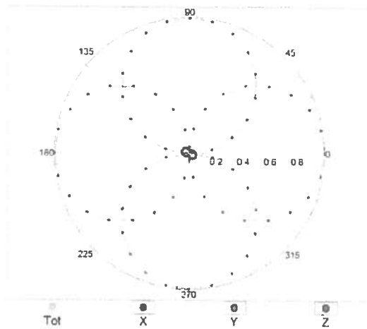
f=2500 MHz,R22,0°
