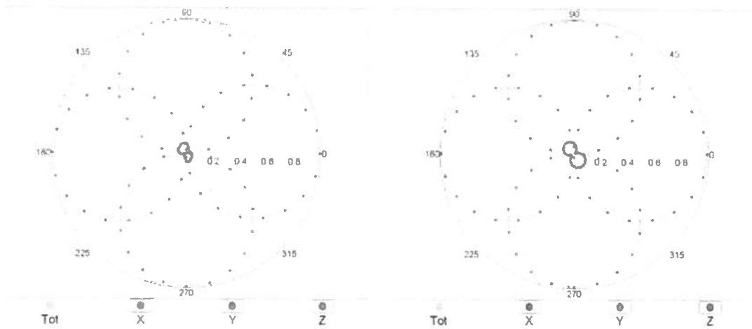
f=2500 MHz, R22, 0^\circ
