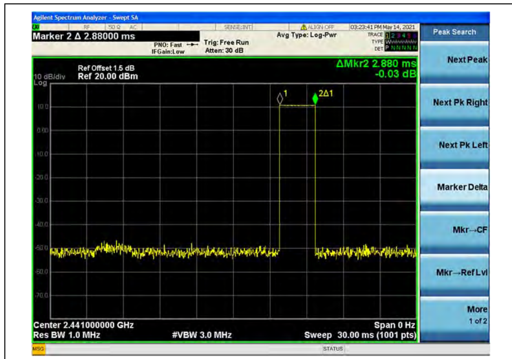
(DH5, 8-DPSK)
