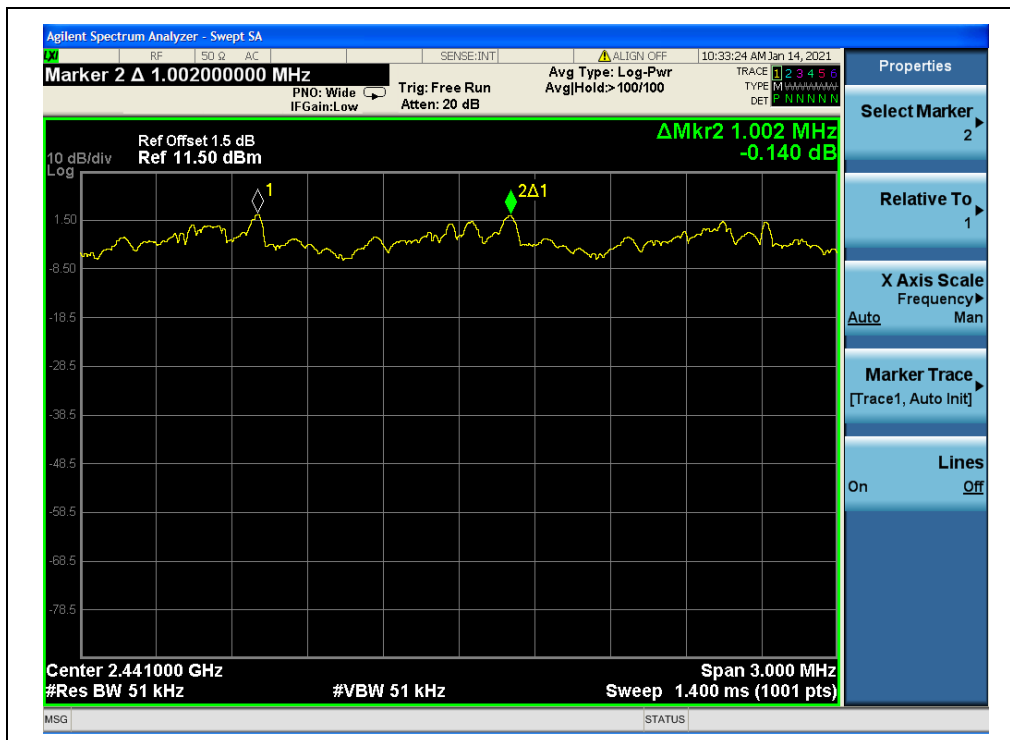
(8-DPSK)
