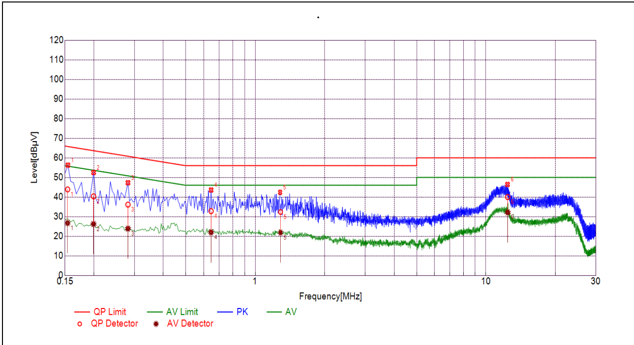
(N Phase)
