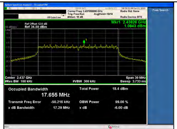
11n-20MHz-6dB BW-Mid-MCS7
