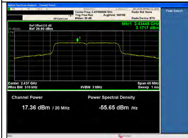
11n-20MHz-PWR-Mid-MCS0
