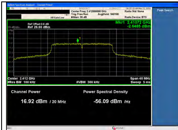
11n-20MHz-PSD-Low-MCS0
