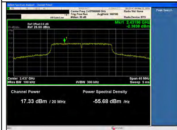
11n-20MHz-PSD-Mid-MCS0
