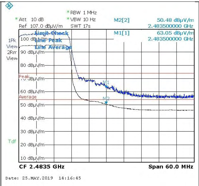
802.11n 2462M--High
