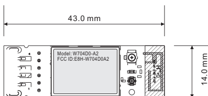
Top Side
