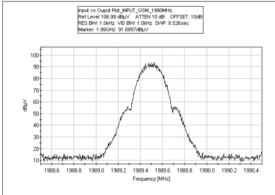
GSM – 1990 MHz Input
