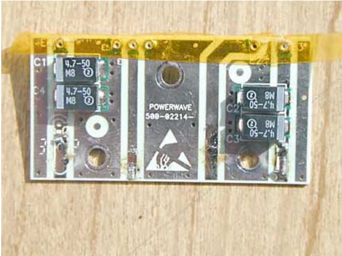
500-02214 PCB top
