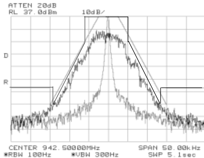
Mask per 101.111(5) & RSS-119 (Mask D)
