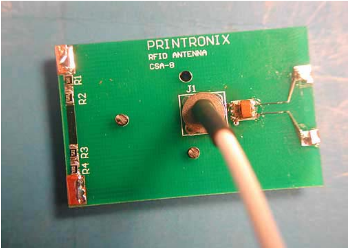
Ant Back
