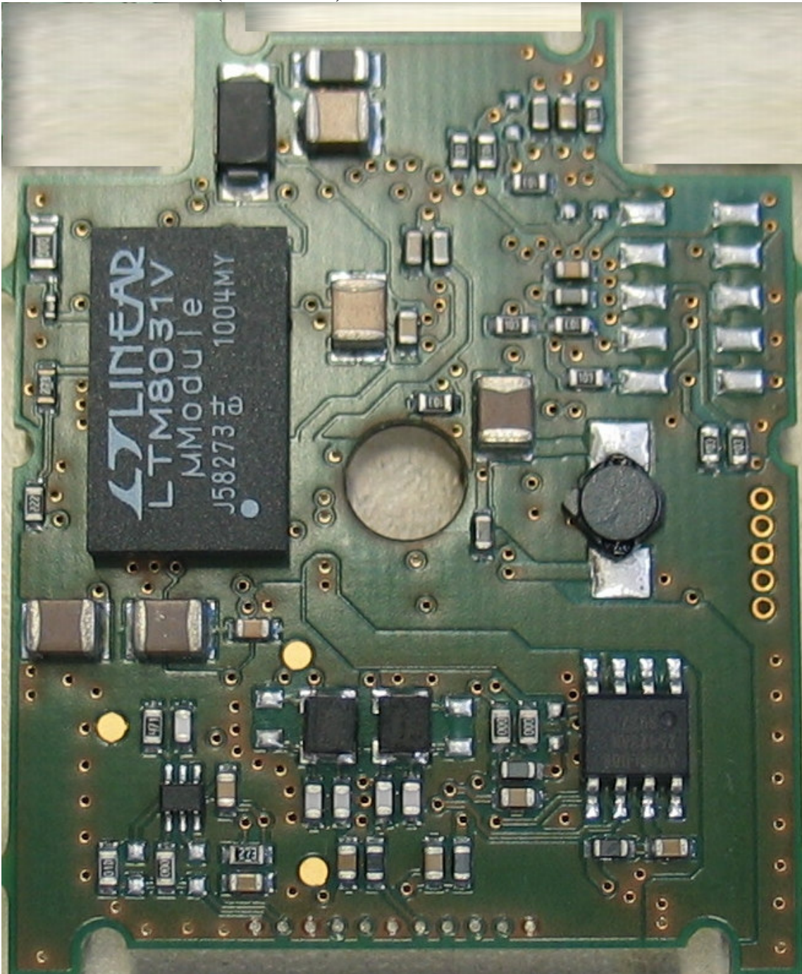
GEL-3440 MAIN 232 ( BOTTOM )
