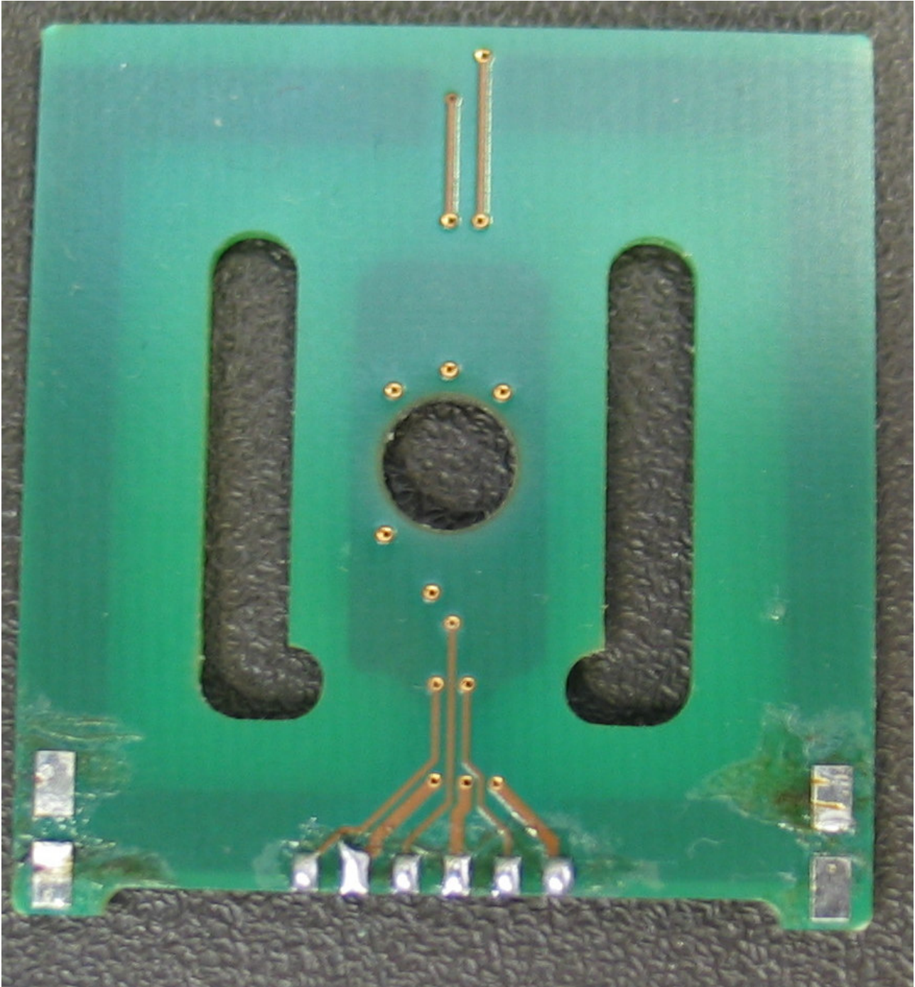
GEL-3251 ANTENNA ( BOTTOM )
