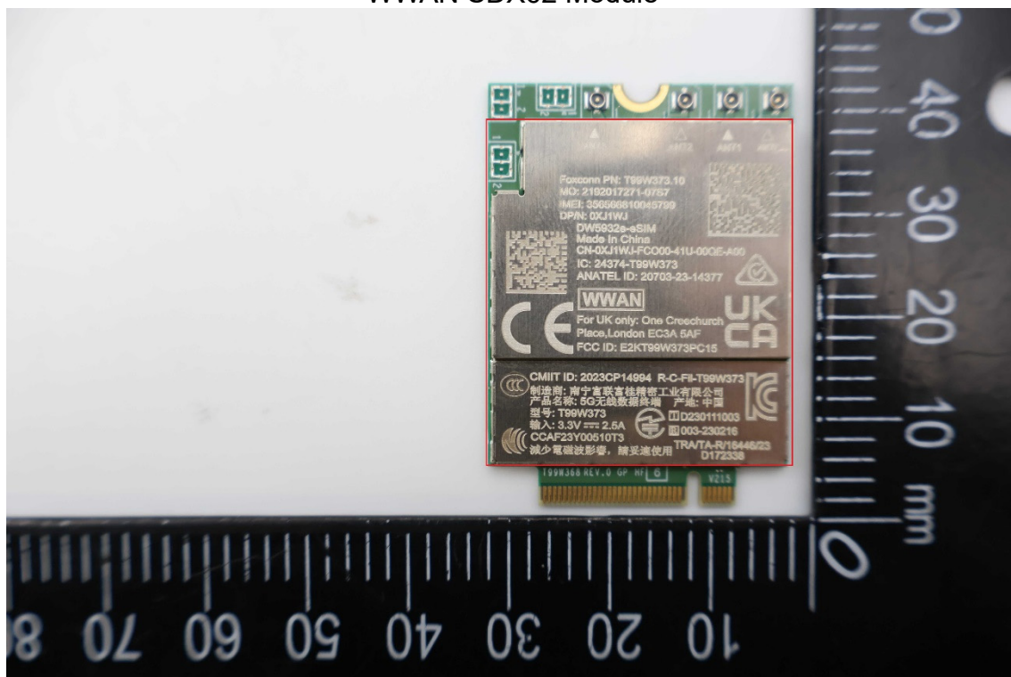
WWAN SDX62 Module
