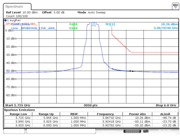
BE-NR-HIGH, SISO-B, 802.11ax20-HE0, Ch173
