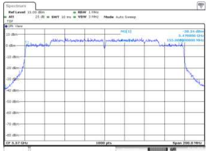
SISO A, CH114, 802.11ax160, HE0, 99%
