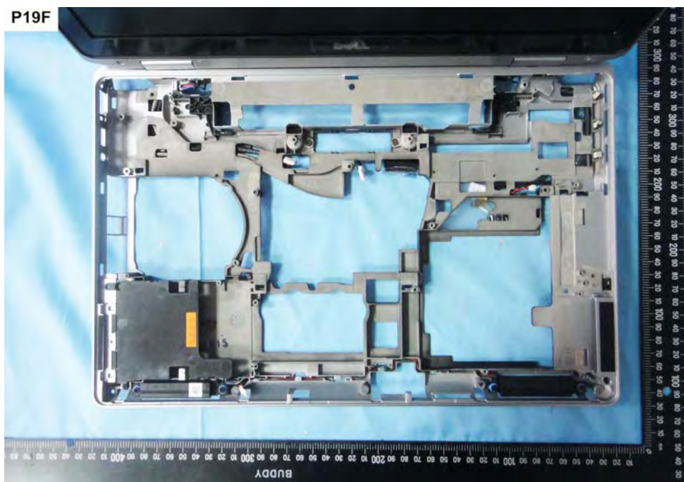
EUT Photo 96 )
