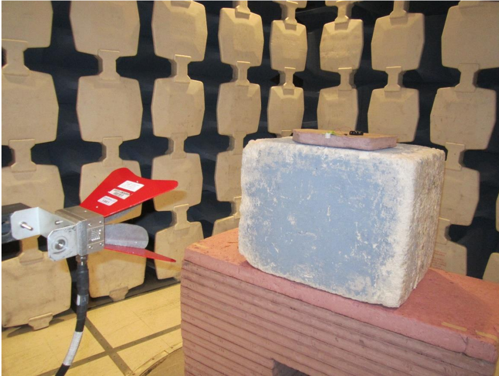
6-18GHz
