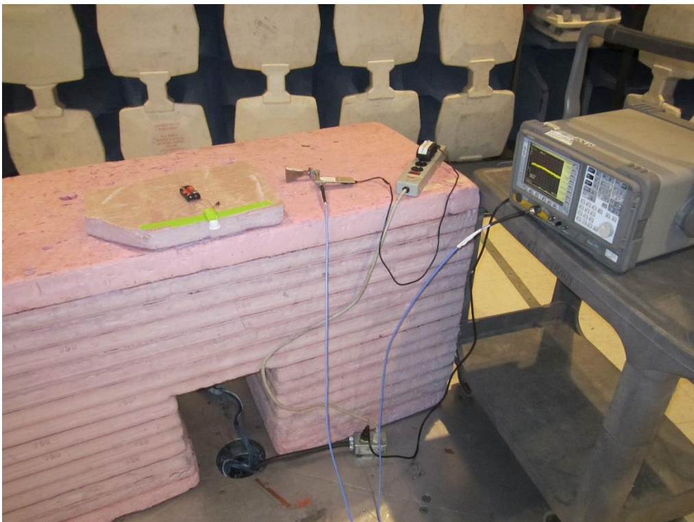
18-25GHz
